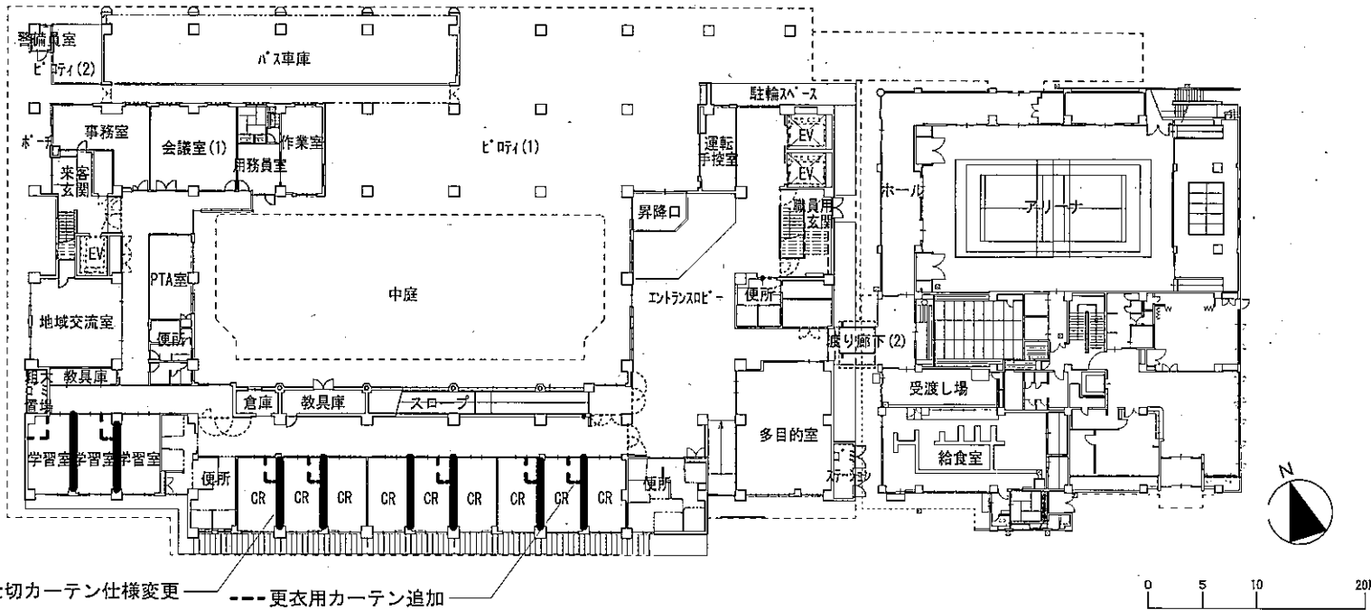
1階平面図
