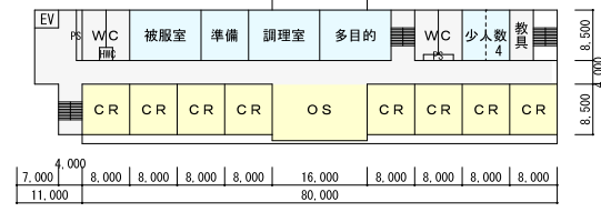
4階平面図 1/1000
