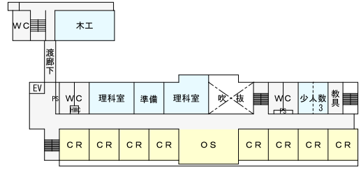
3階平面図 1/1000
