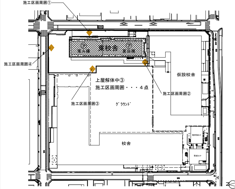
測定計画図 上屋解体中③ (6/23)
