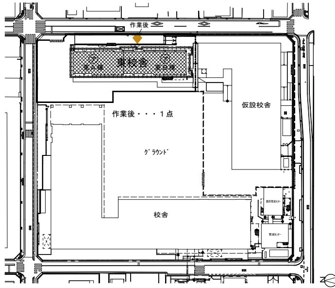
測定計画図 上屋解体中② (6/16)
