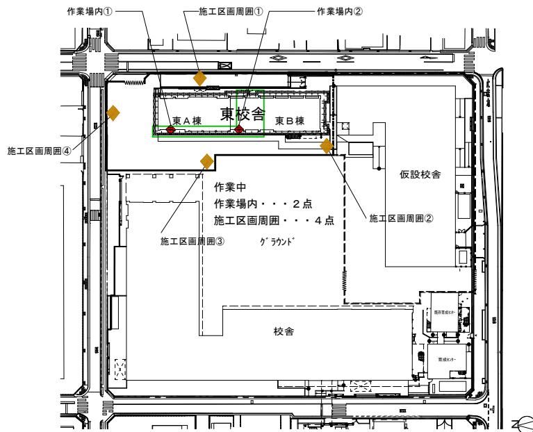
測定計画図 作業中③ (5/17)
