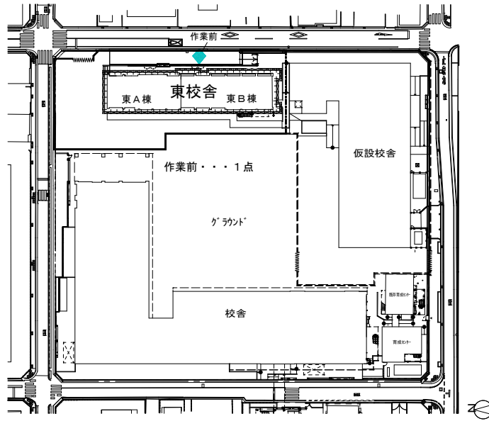
測定計画図 作業前 (4/19)
