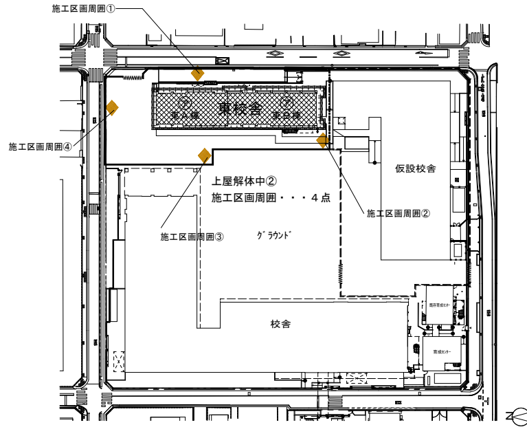
測定計画図 上屋解体中② (6/16)
