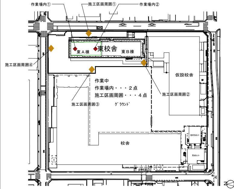
測定計画図 作業中① (4/25)
