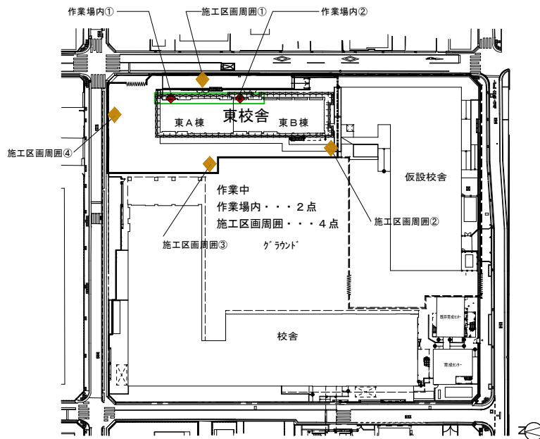
測定計画図 作業中② (5/2)
