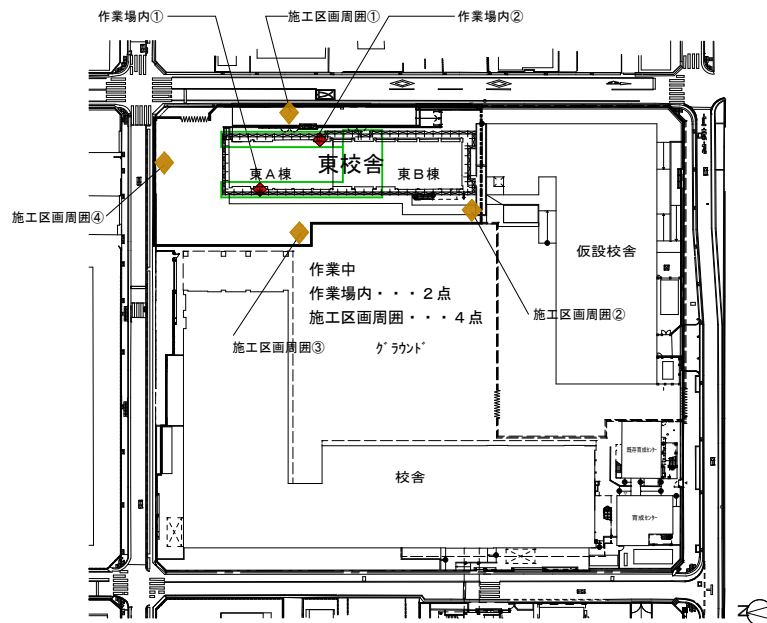
測定計画図 作業中②③ (5/11)
