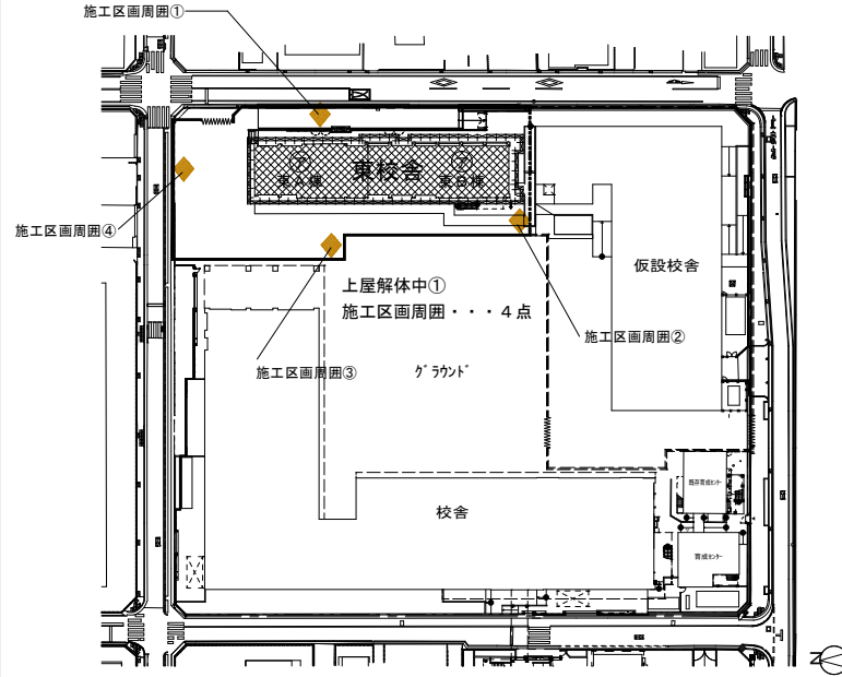
測定計画図 上屋解体中① (6/9)
