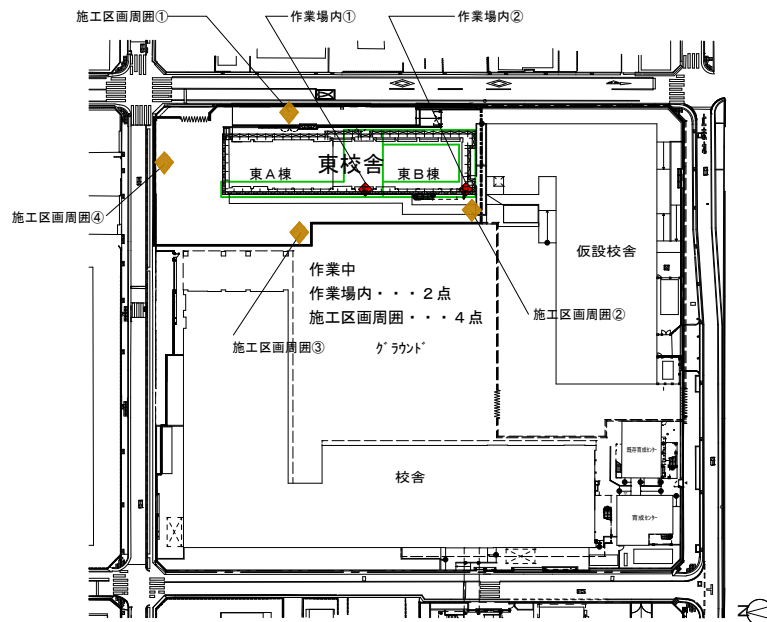
測定計画図 作業中③④ (5/23)
